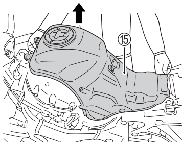
14. 拆卸油箱 ⑮。
