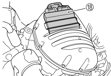
17. 拆卸鬆緊帶。從空氣濾清器蓋取下 ECM ⑱。
