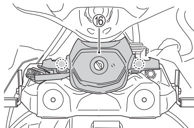
15. 卸離扣鉤，並拆下油箱下蓋總成 ⑯。
