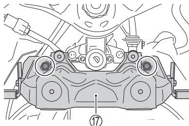
16. 拆下螺栓並取下油箱支架 ⑰。
